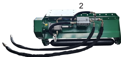
1 = drænslange (retur slange) 2 = tilslutning til olieventil køretøj
