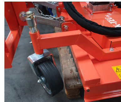
Justerbar højdehjul foran klipperen
